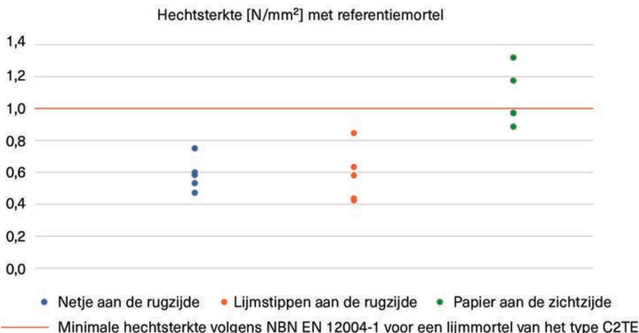
Abbeelding 3: Resultaten van de hechtproeven op mozaïekelementen met drie verschillende assemblagewijzen.
