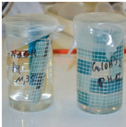
Afbeelding 2: Proef op de duurzaamheid van de verlijming van mozaïeken op net.
